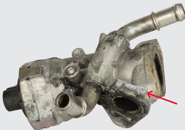
Motore/solenoide mancante
