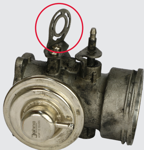
Componente mancante
